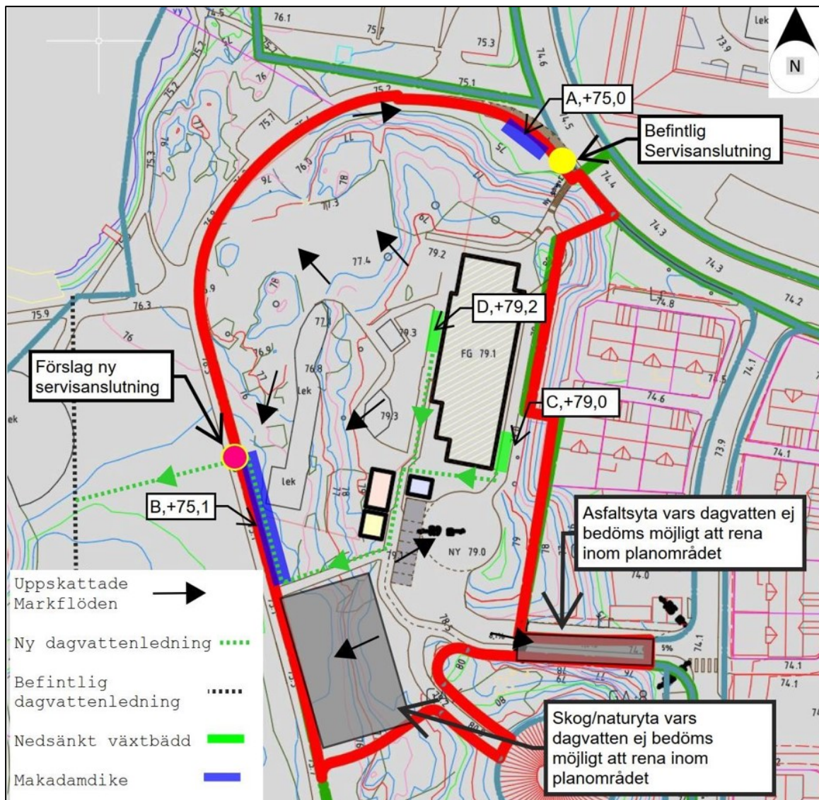
Förslag på placering av åtgärder för fördröjning och enklare rening
